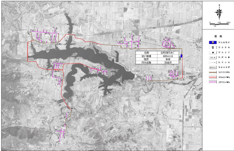
石舌镇规划污水处理设施及管网分布图
